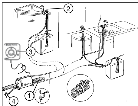
Schema van de watervoorziening
