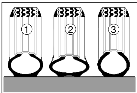
Verschillende luchtdrukken van de banden
